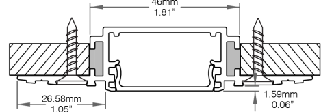
Vue Sectionnelle
