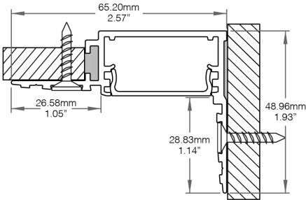
Vue Sectionnelle
