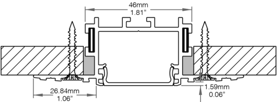
Vue Sectionnelle
